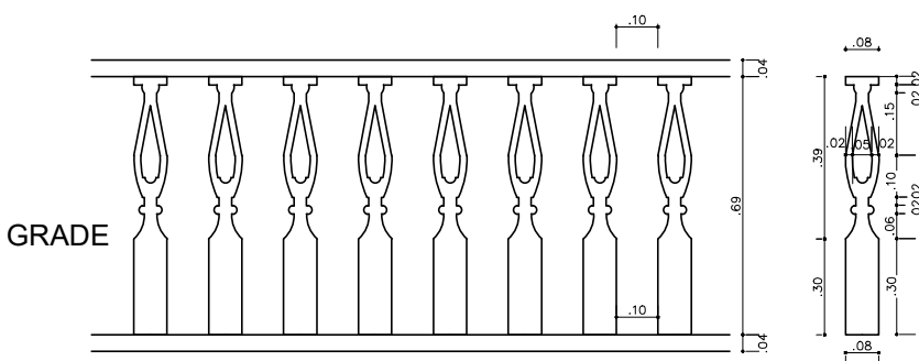
DETALHE GRADIL
