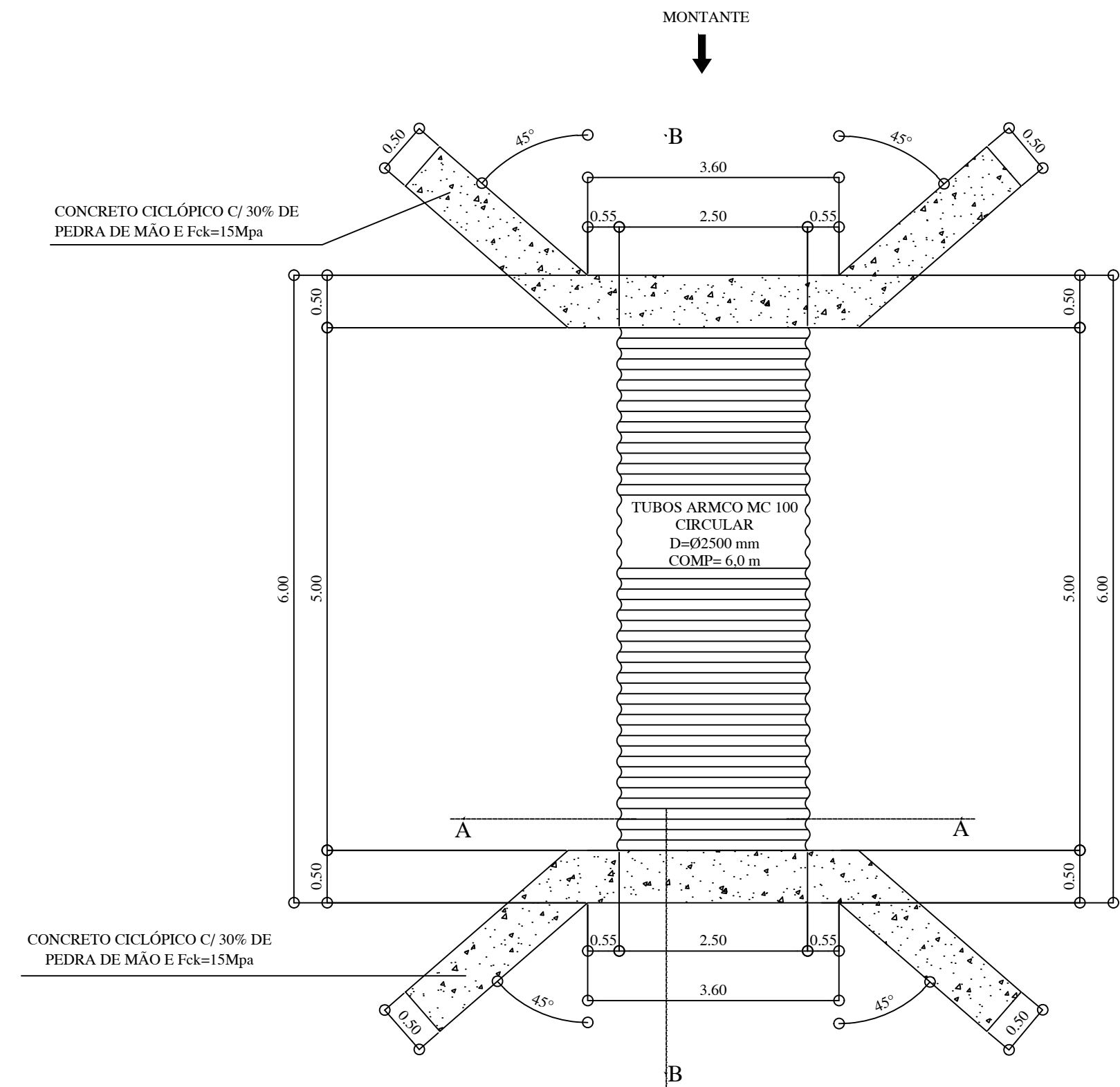
1 PLANTA DE IMPLANTAÇÃO ESCALA 1:50
